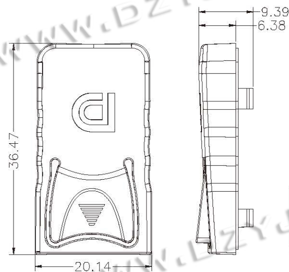
上盖
