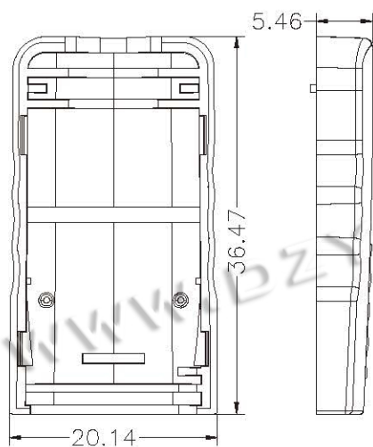
下盖
